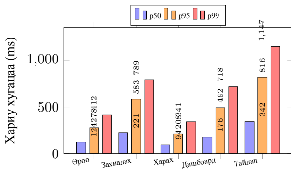
Зураг 7: Ачааллын туршилтын endpoint хариу хугацаа (ms)
