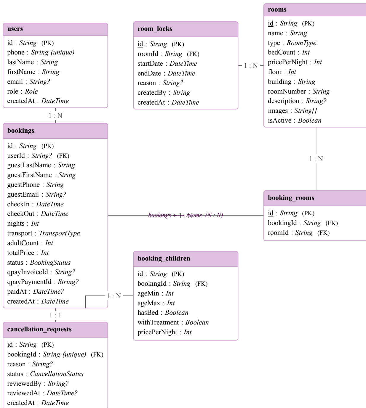
Зураг 3.9: Өгөгдлийн сангийн ER диаграмм
