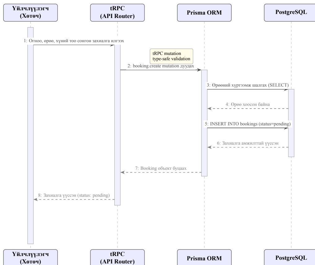
Зураг 3.7: Захиалга үүсгэх дараалал диаграмм
