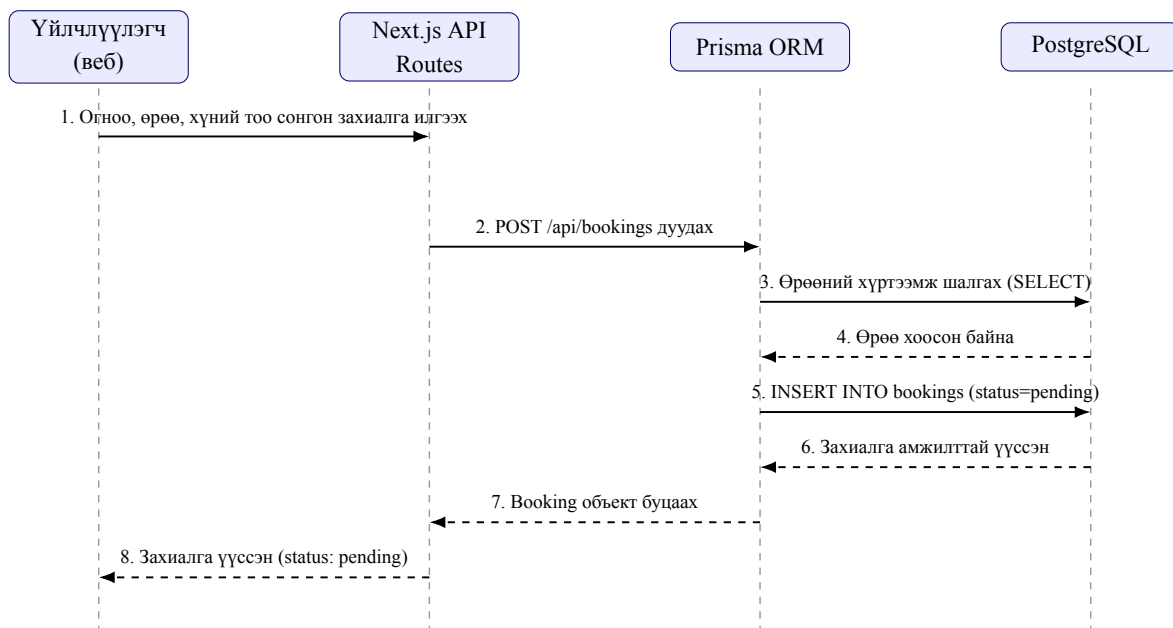
Зураг 3.8: Захиалга үүсгэх дараалал диаграмм
