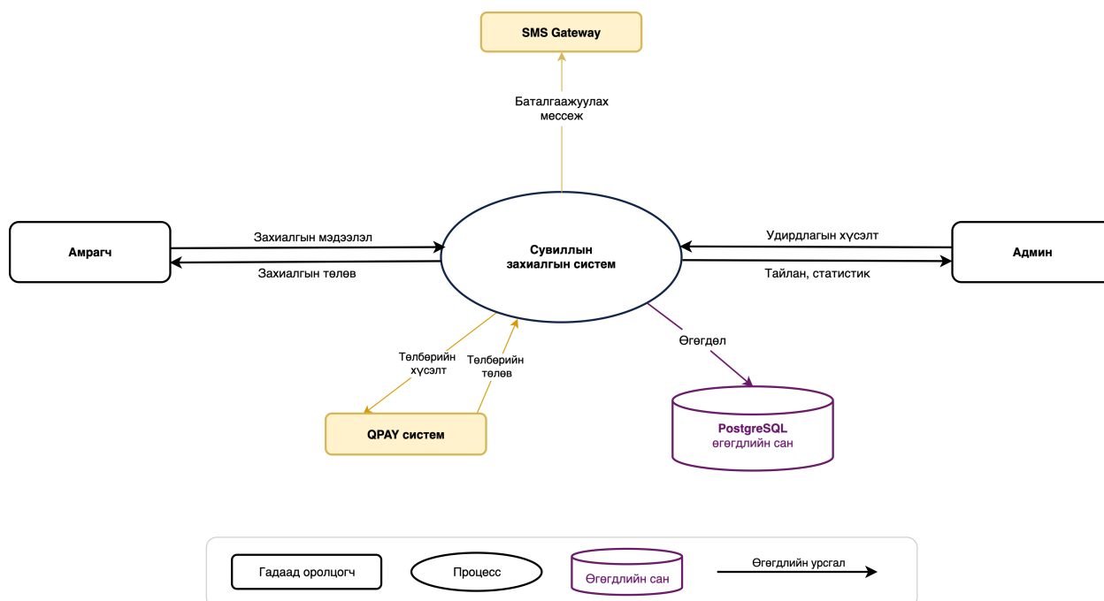
Зураг 3.2: Сувиллын захиалгын системийн өгөгдлийн урсгалын диаграмм
