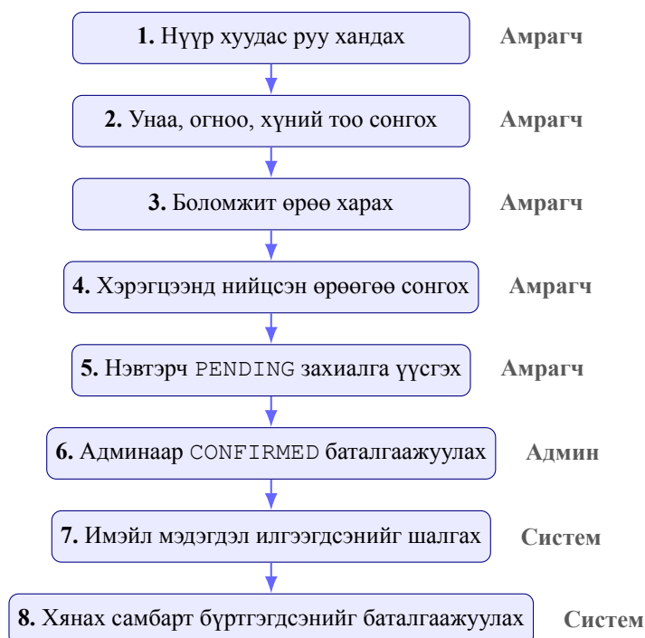
Зураг 3.15: E2E туршилтын 8 алхамт урсгал
