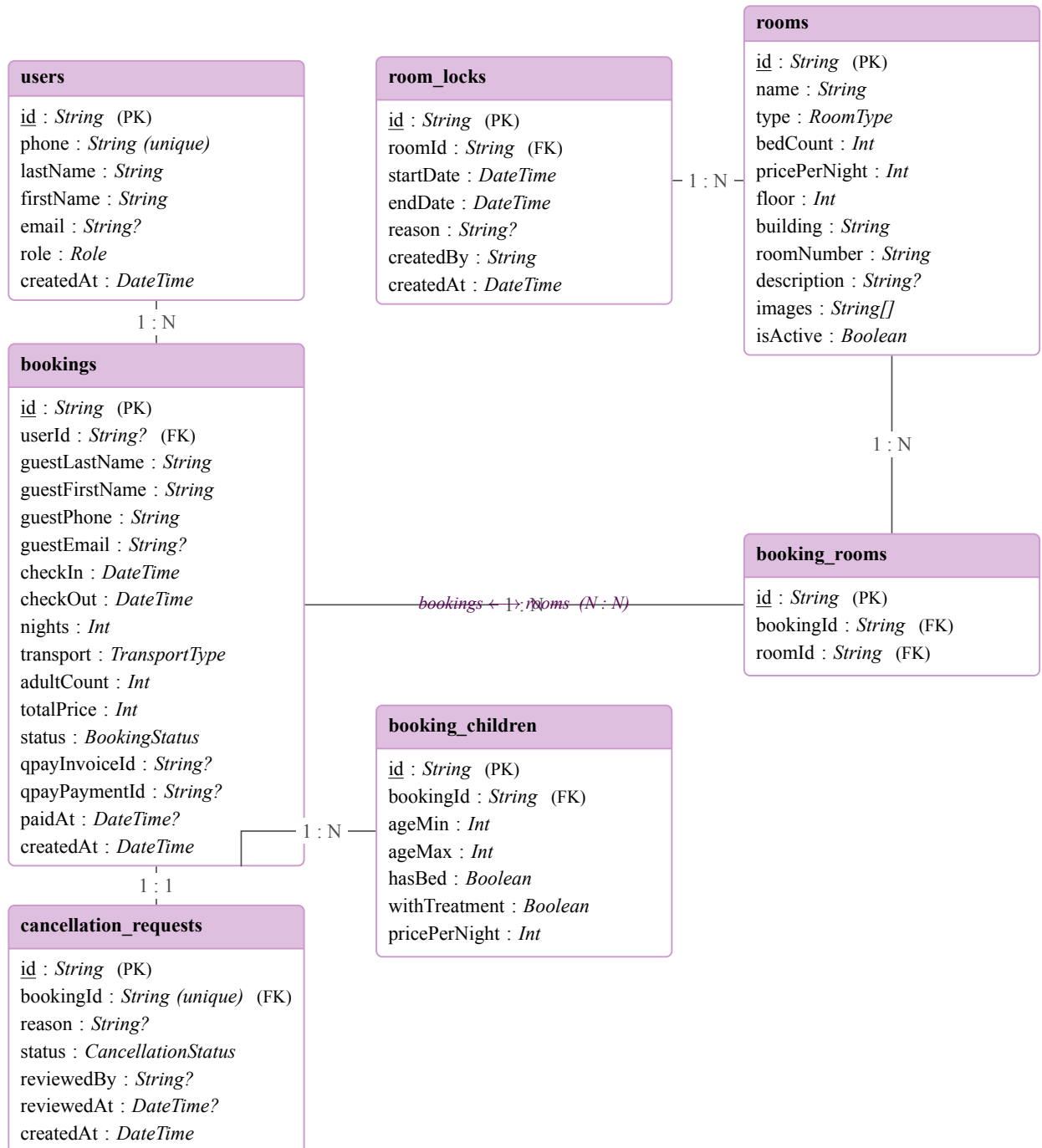
Зураг 3.10: Өгөгдлийн сангийн ER диаграмм
