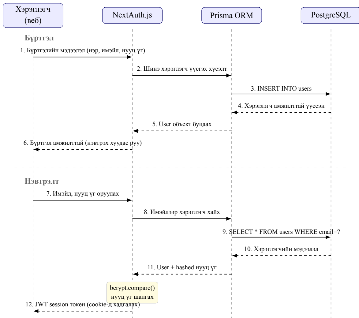
Зураг 3.7: Бүртгэл ба нэвтрэлтийн дараалал диаграмм
