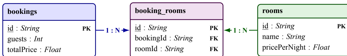
Зураг 3.11: bookings ба rooms хоорондын N:N харилцааны загвар
