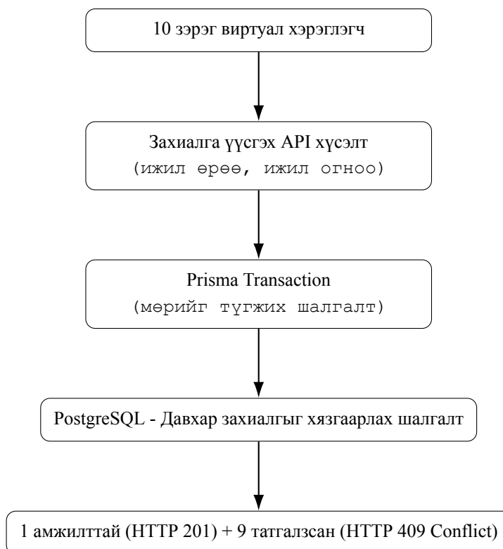
Зураг 3.12: Зэрэг захиалгын туршилтын өгөгдлийн урсгал
