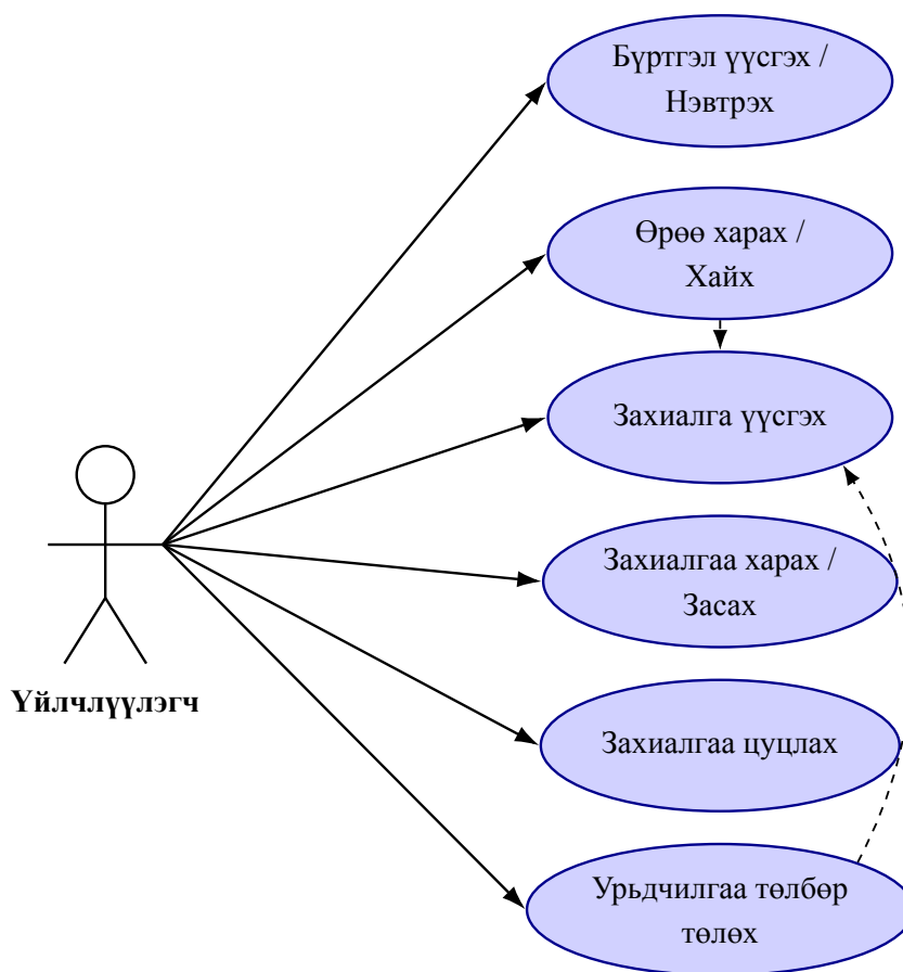
Зураг 3.5: Үйлчлүүлэгчийн юзкейс диаграмм
