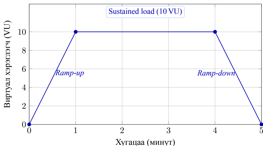
Зураг 3.13: k6 ачааллын туршилтын ramp-up стратеги (5 минут, 10 VU)
