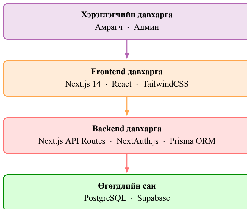
Зураг 3.1: Системийн дөрвөн давхаргат архитектур
