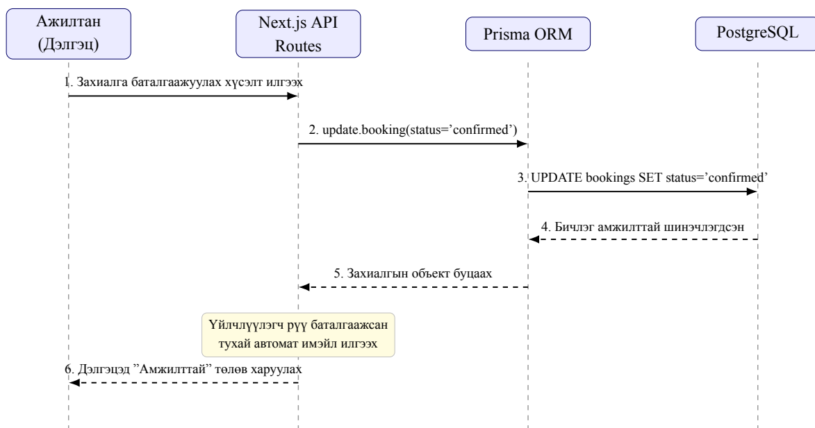
Зураг 3.9: Захиалга баталгаажуулах дараалал диаграмм
