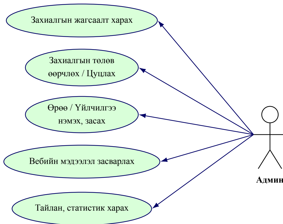
Зураг 3.6: Админы юзкейс диаграмм
