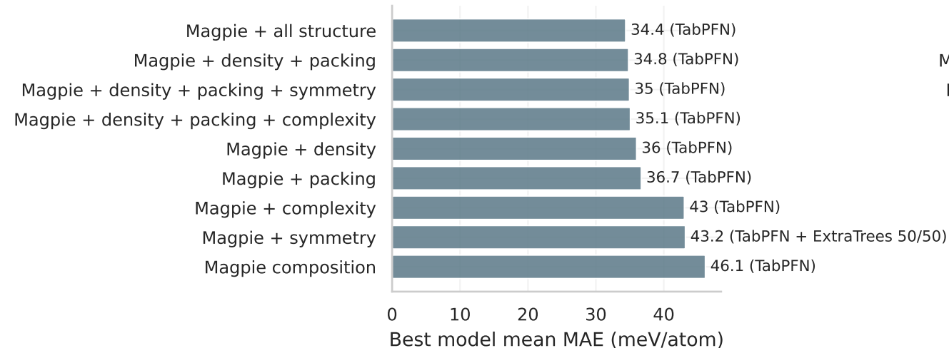
matbench_jdft2d
