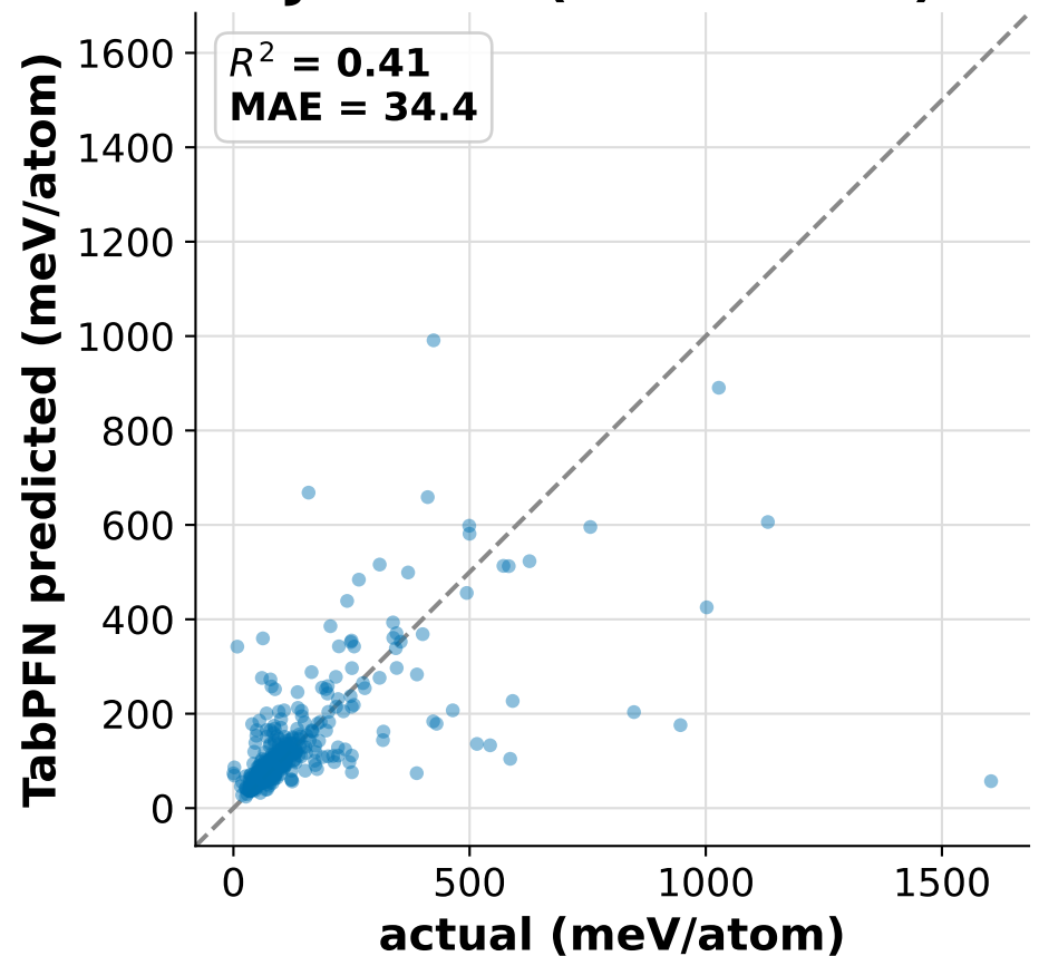
JDFT2D (+ structure)
