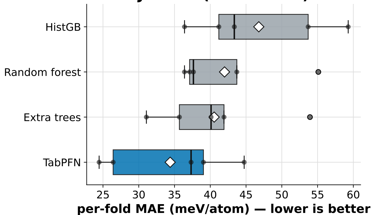
JDFT2D (+ structure)
