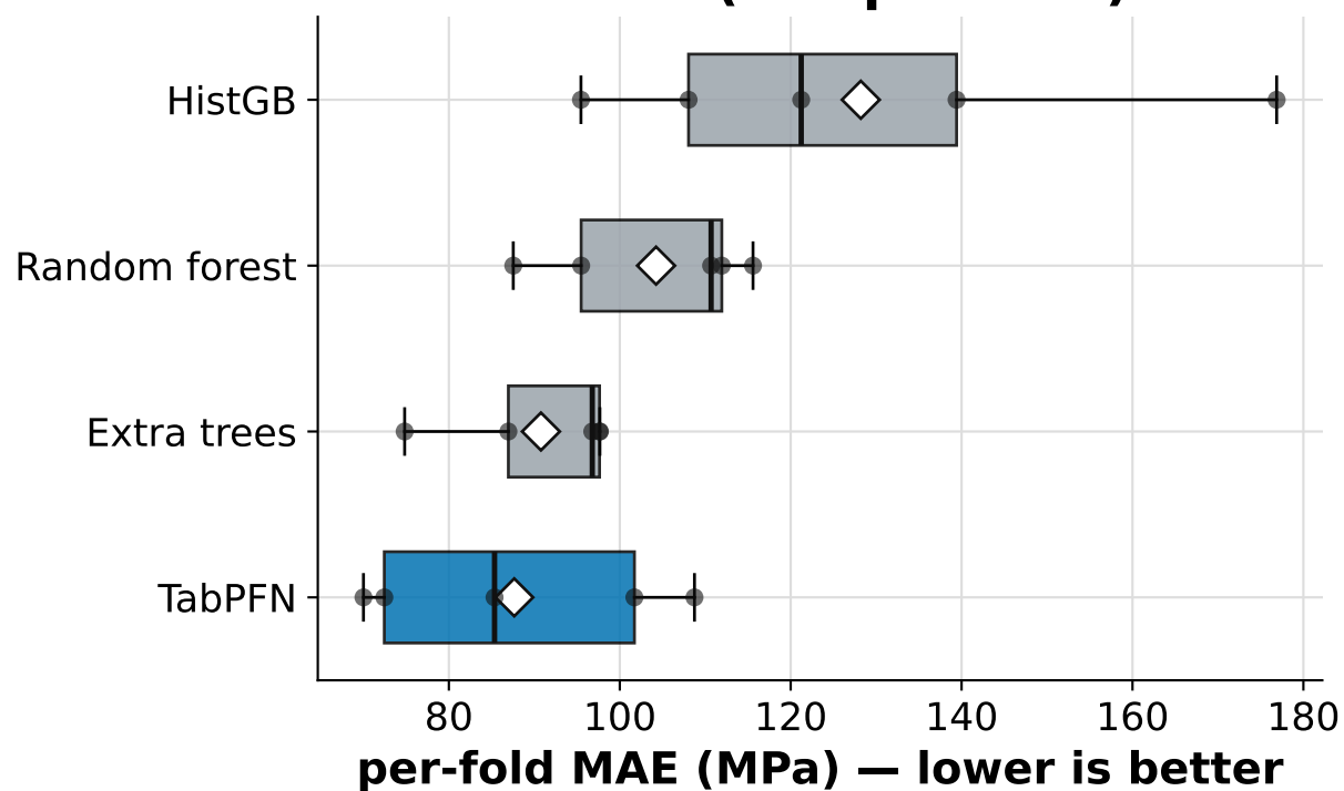
JDFT2D (+ structure)
