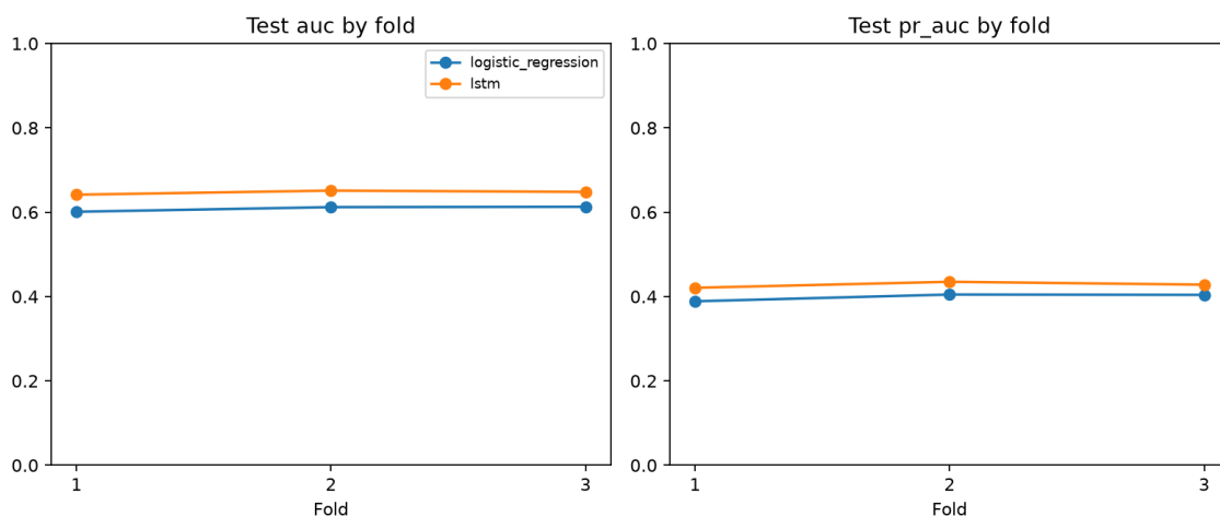
图 7.3: 三折walk-forward 的逐折指标。逐折结果可用于判断表现是否集中在某一时间窗口。
