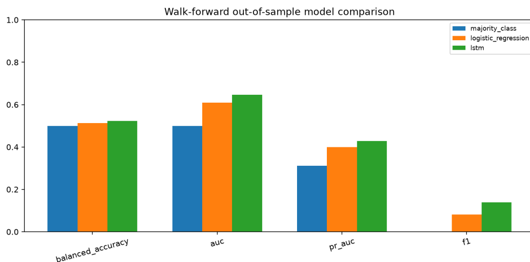
图 7.1: 多数类、逻辑回归和LSTM 的样本外指标比较。LSTM 的排序指标高于逻辑回归。
