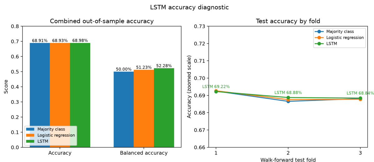
图 7.1: LSTM 准确率诊断。左图比较合并样本外Accuracy 与Balanced Accuracy; 右图比较三折测试Accuracy。由于类别不平衡, 总体Accuracy 必须与多数类基线、平衡准确率和排序指标一起解释。
