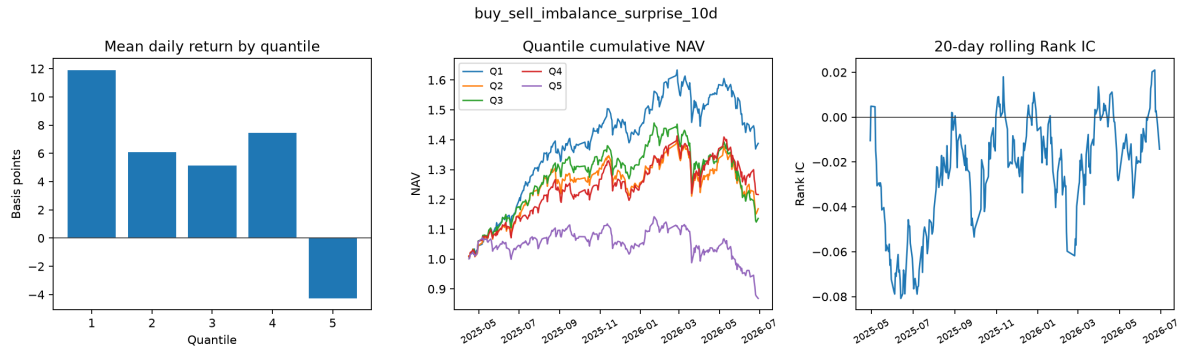
图 4.2: 主动买卖不平衡冲击因子诊断。Rank IC 为-0.0251, 原始Q5-Q1 为-37.95%; 按负向因子构造Q1-Q5 后累计多空收益为59.07%, 体现订单流异常后的短期反转。
