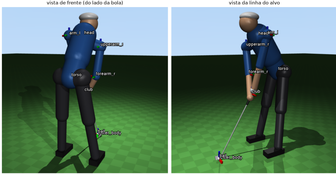
Figura 1: Referenciais dos corpos na pose de endereço ( q = 0 ): vermelho x , verde y , azul z . Nesta pose todos coincidem em orientação com o referencial do mundo, cuja origem está na bola.
