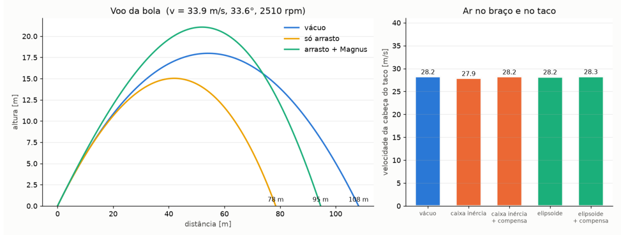
Figura 4: Esquerda: voo da bola com as condições de saída do swing, no vácuo, só com arrasto e com arrasto + Magnus. Direita: velocidade da cabeça do taco com três modelos de ar no braço e no taco, com e sem compensação do arrasto pelo controlador.
