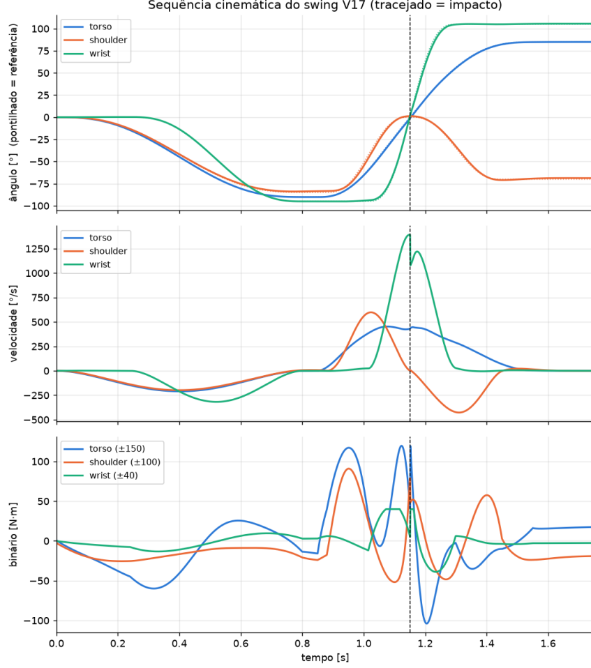
Figura 3: Ângulos, velocidades e binários das três juntas atuadas.
