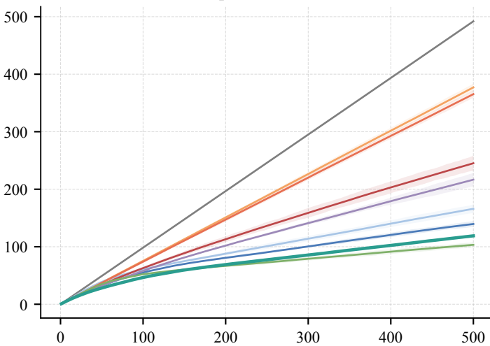
DeepSeek-V4-Flash
