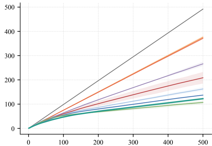
GPT-5.2
