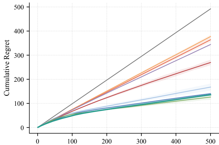
Qwen3-30B
