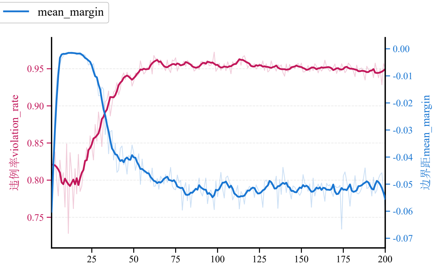
(b) CiteSeer
