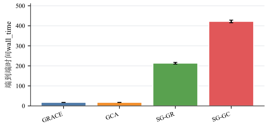
(d) DBLP
