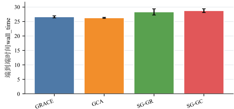
(b) CiteSeer
