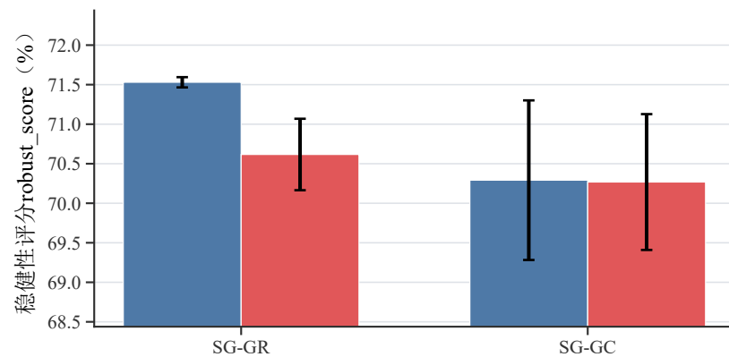
(d) DBLP
