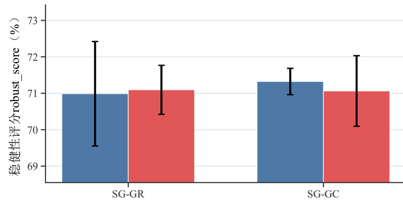
(b) CiteSeer
