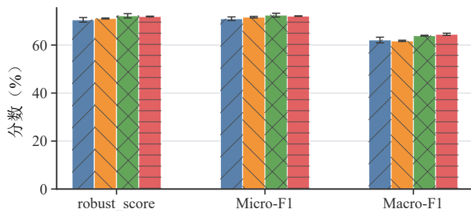
(d) DBLP
