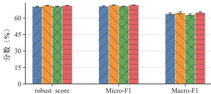
(b) CiteSeer
