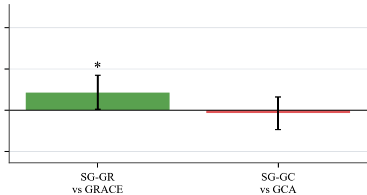
(d) DBLP
