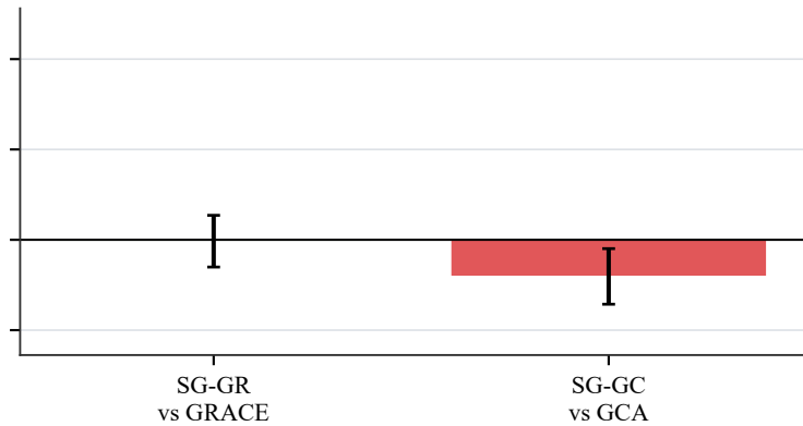
(b) CiteSeer
