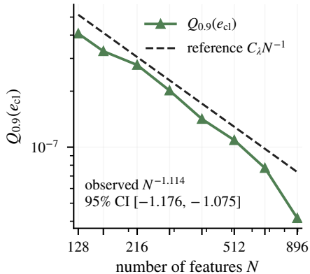
(b) Eigenvalue error
