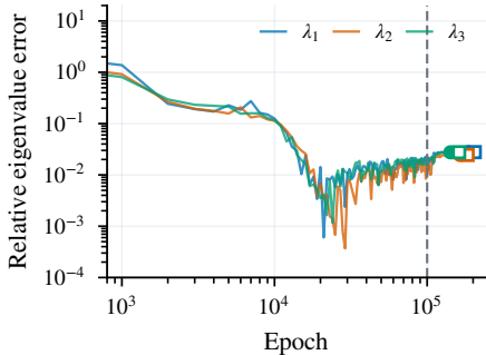
(b) 10D DRM: V(t) = e^{-\pi t}
