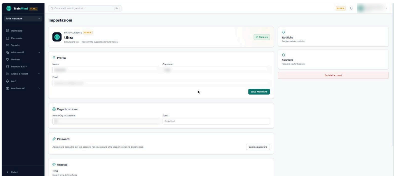
Figura 18.1 — Impostazioni
