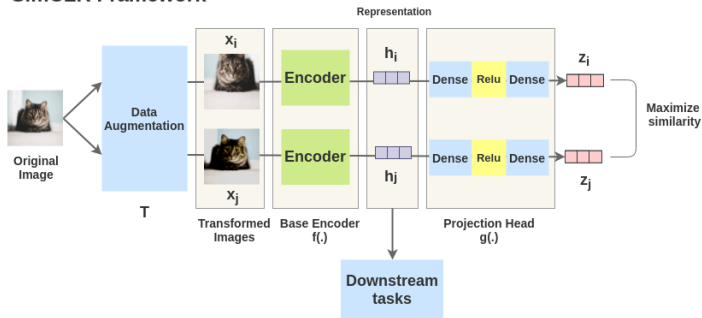
SimCLR Framework
