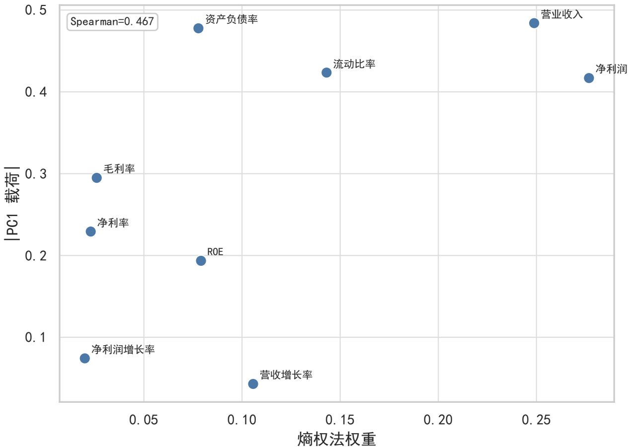
熵权与 PCA 载荷对比：规模利润指标在两种方法中都靠前
