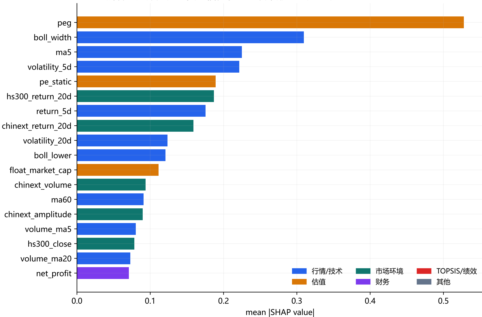
SHAP 解释：短期方向主要由估值状态与技术形态共同驱动
