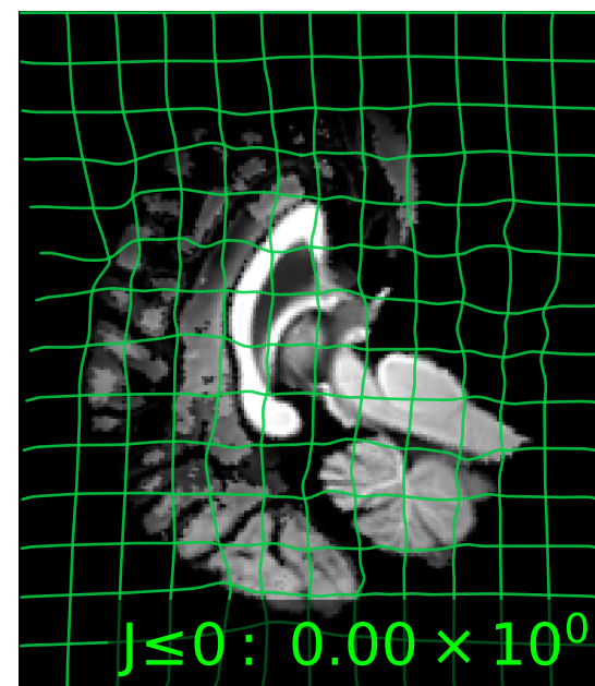
MIDIR
