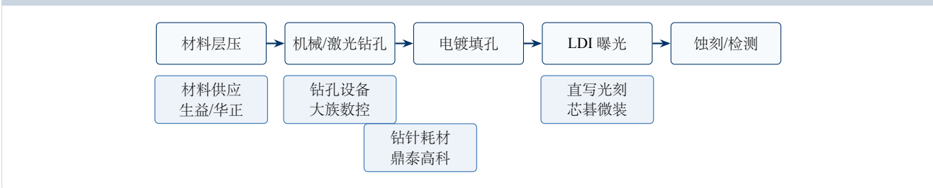
图表 3-8：PCB 制造流程与材料/设备/耗材映射
