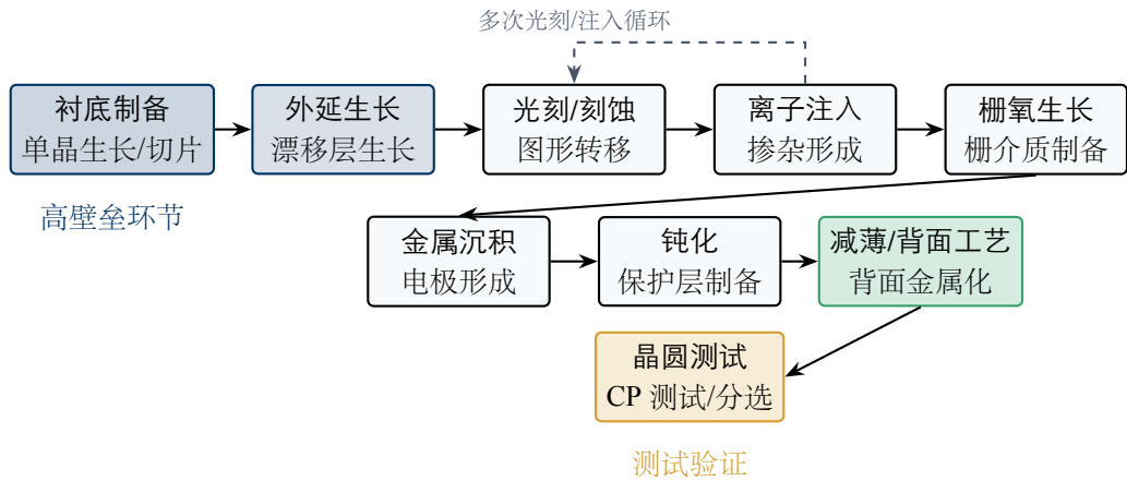
图 4-4：功率半导体晶圆制造工艺流程
