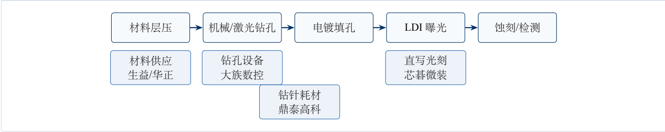
图表 3-10：PCB 制造流程与材料/设备/耗材映射
