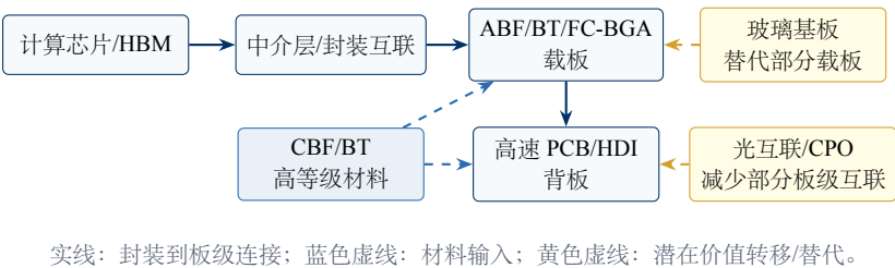
图表 3-9：先进封装与载板材料关系
