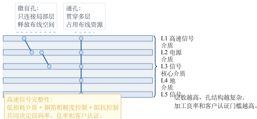
图表 3-5: HDI 与高多层板层叠示意
