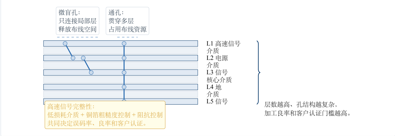
图表 3-5：HDI 与高多层板层叠示意
