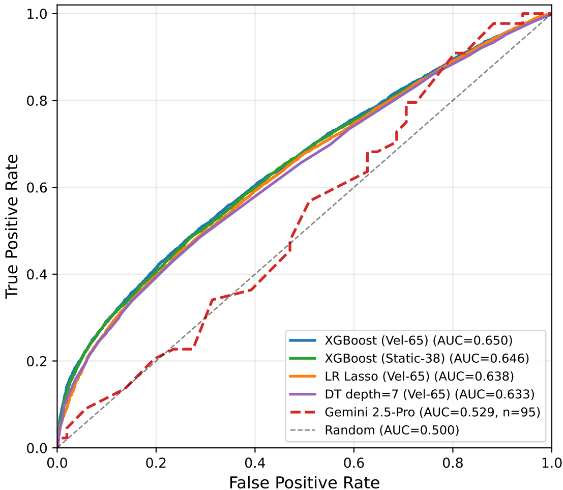
ROC Curves — Tabular Baselines
