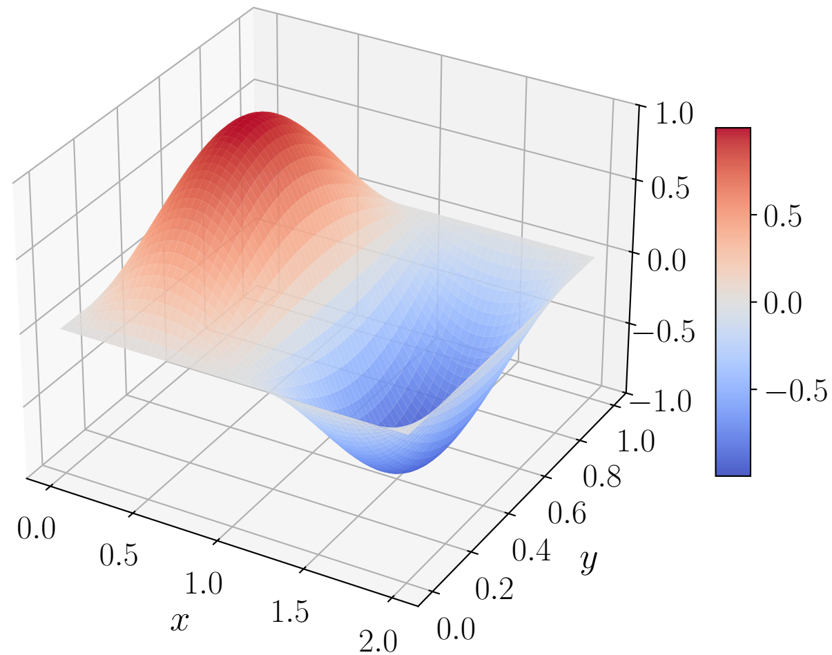
Mode m=2 , n=1
