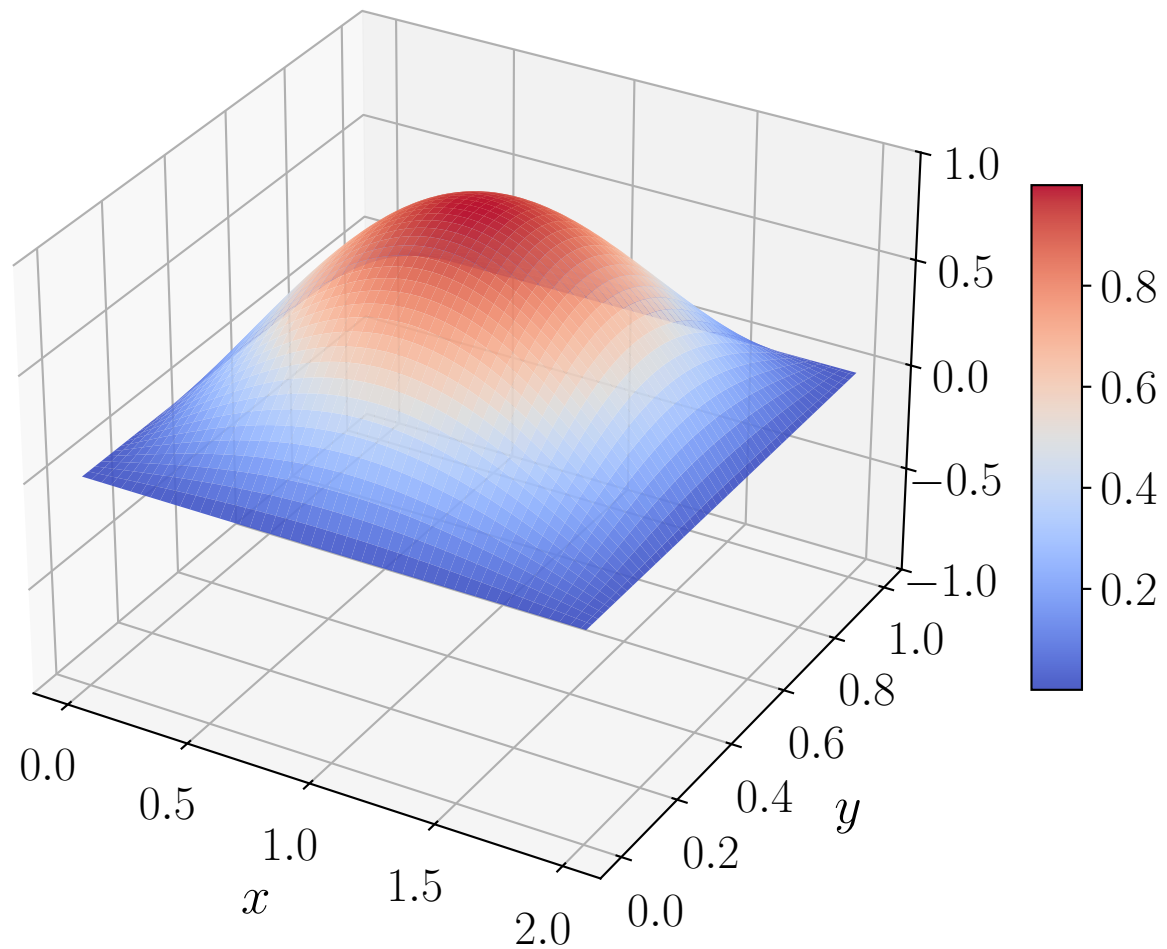
Mode m=1 , n=1
