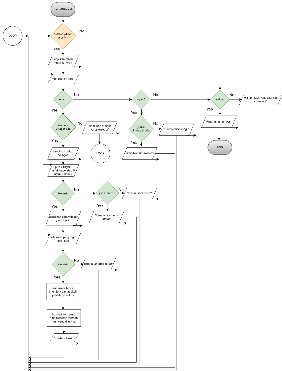
Gambar 1.4 Menu User atau Survival
