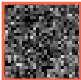
x_t (t=250)
