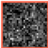
x_t (t=187)
