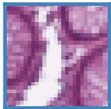
OOD orig.
