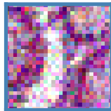
x_t (t=37)
