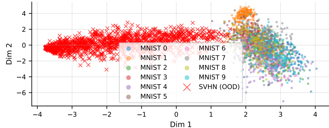
PCA (2D)
