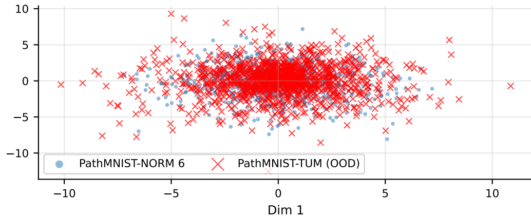
PCA (2D)
