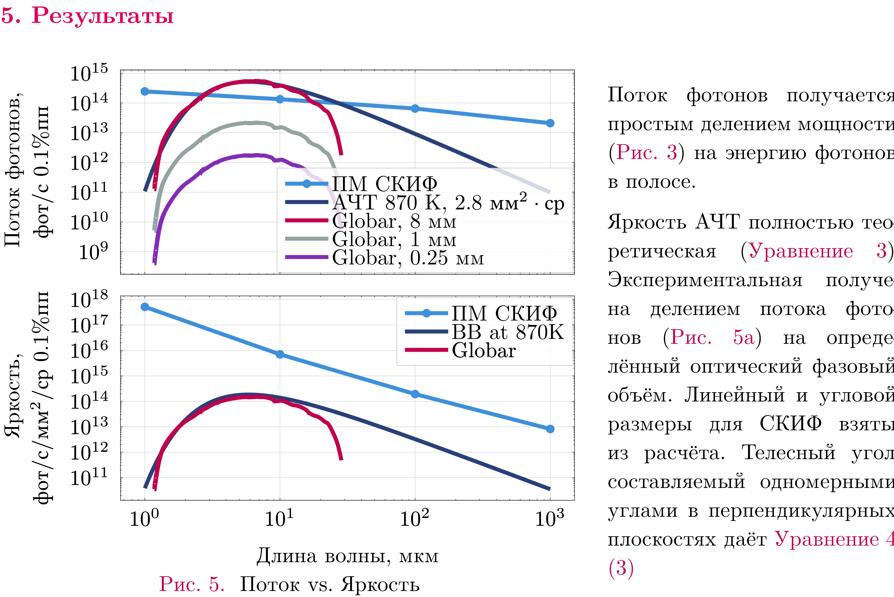
Рис. 5. Поток vs. Яркость
