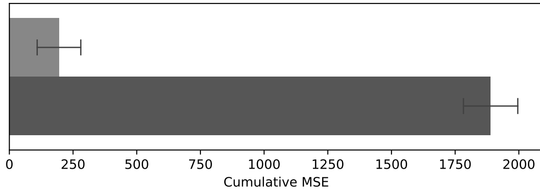
Sinusoid
