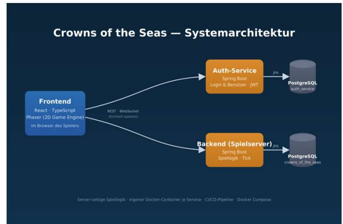
1. Das Frontend kommuniziert per REST und WebSocket mit dem Auth-Service (JWT) und dem Spielservice. Jeder Service läuft in einem eigenen Docker-Container. Der Auth-Service und der Spielservice laufen bewusst getrennt, um Authentifizierung und Spiellogik klar voneinander zu trennen.
