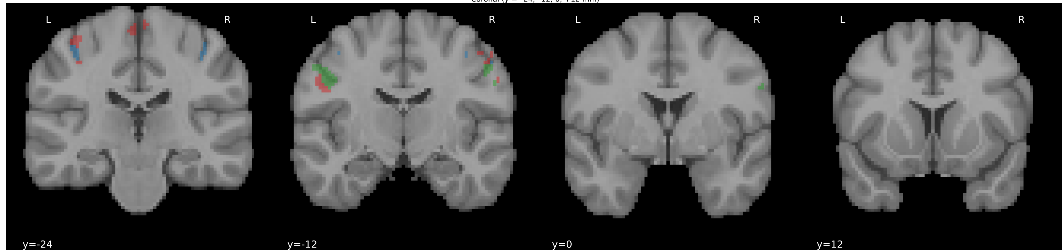
MSC01 — Localizer Sub-Parcel ROI Masks (areas 4 & 3b)
