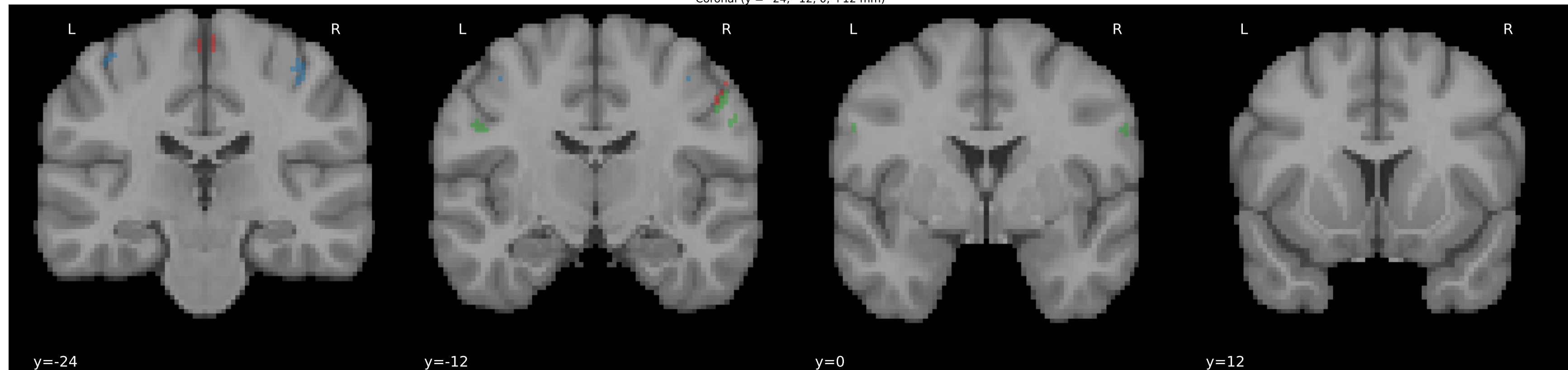
MSC04 — Localizer Sub-Parcel ROI Masks (areas 4 & 3b)
