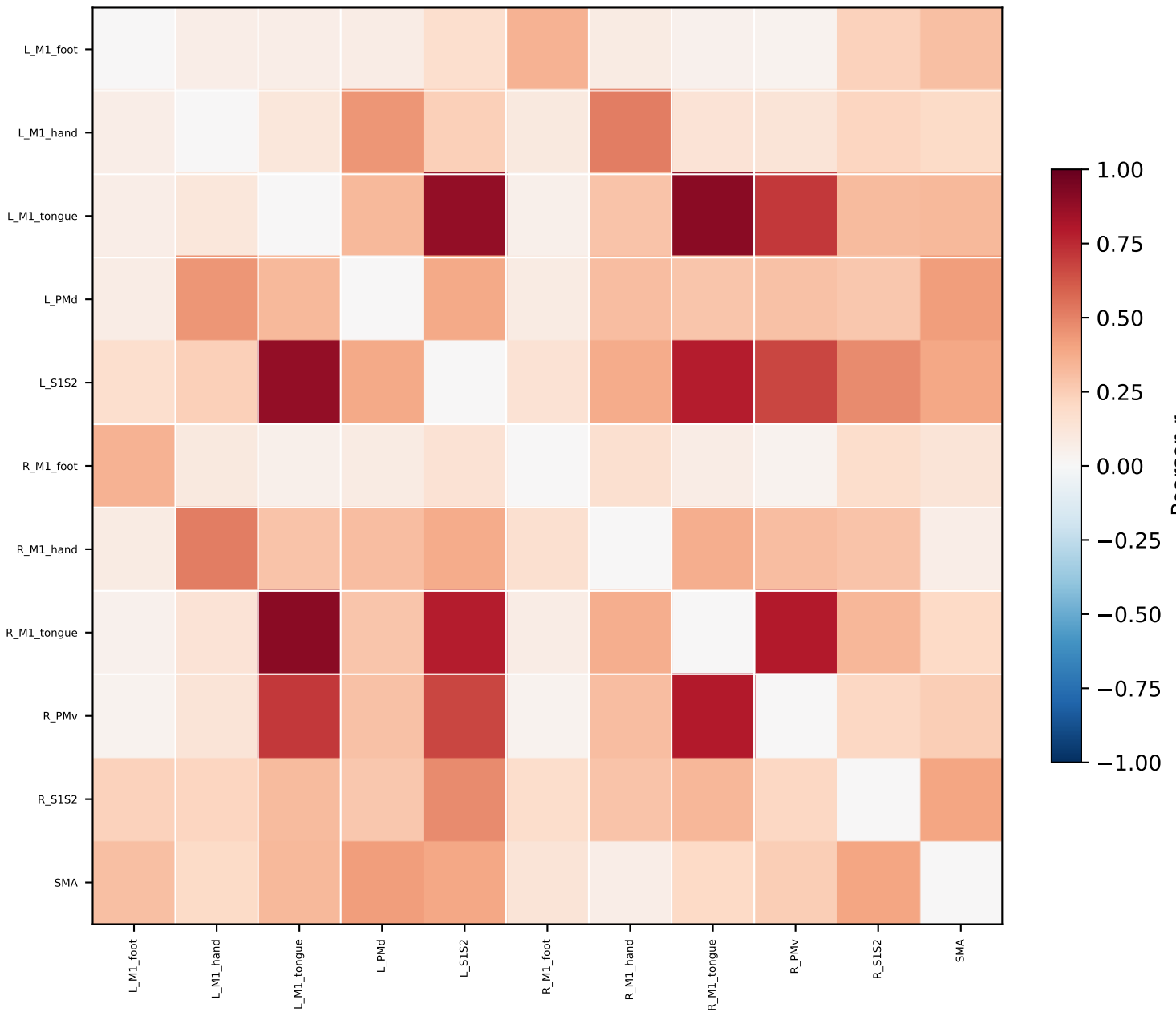
MSC01_func04 — GCSS Motor FC
