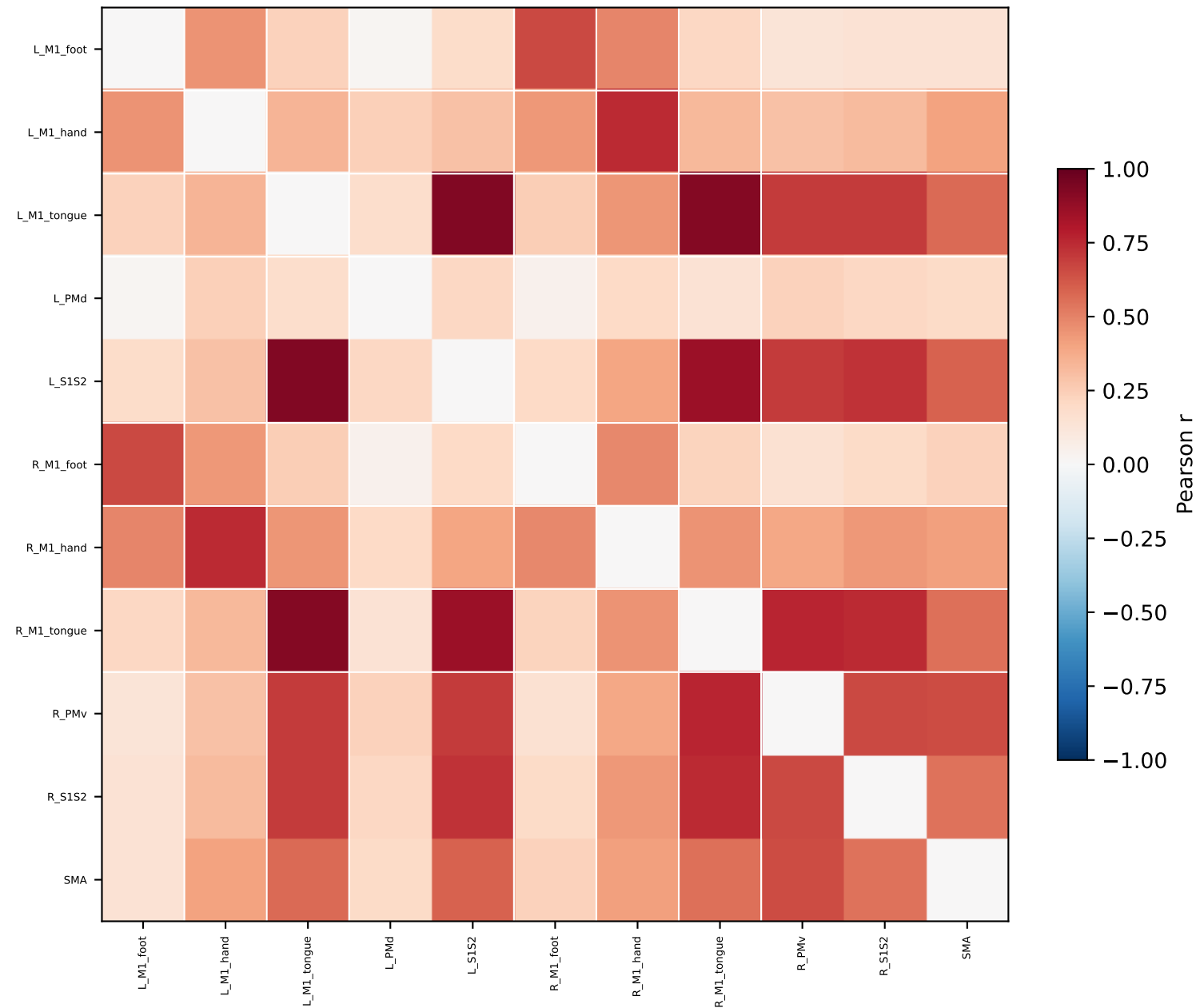
MSC04_func08 — GCSS Motor FC
