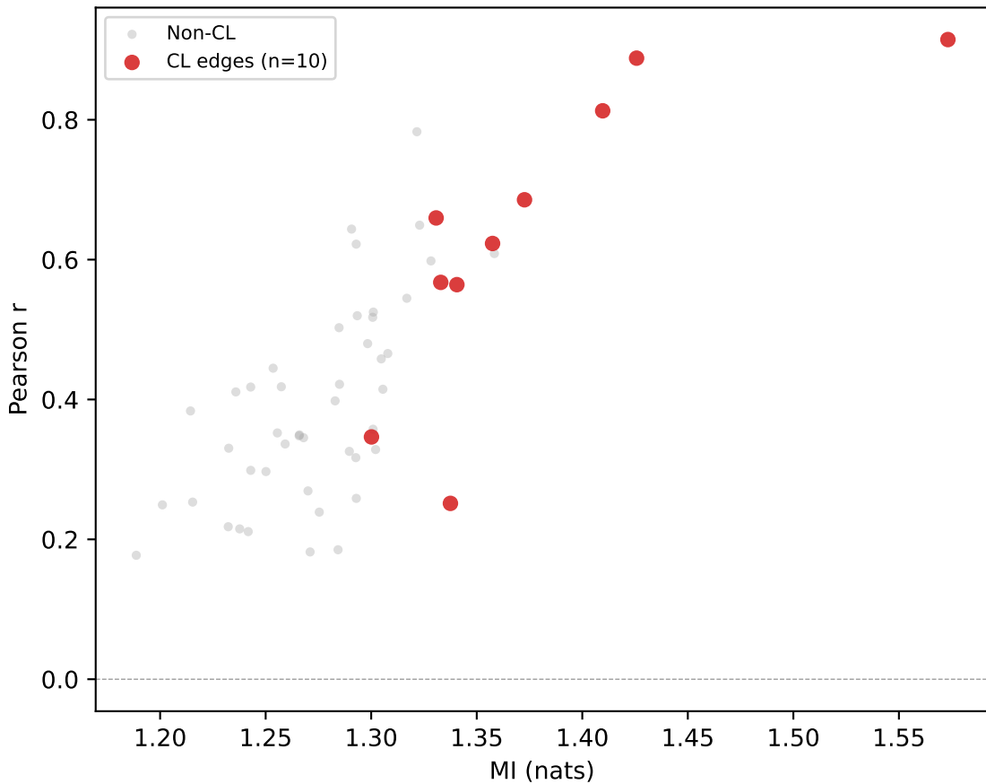
MSC04_func09 — GCSS Motor FC vs MI
