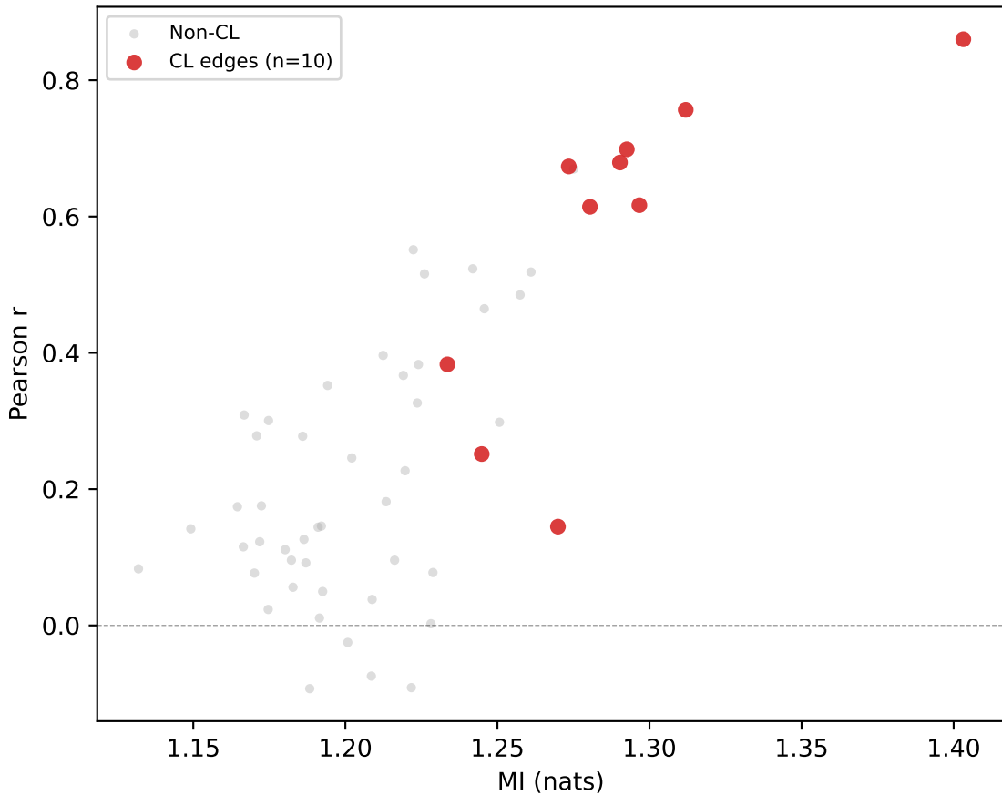
MSC05_func01 — GCSS Motor FC vs MI
