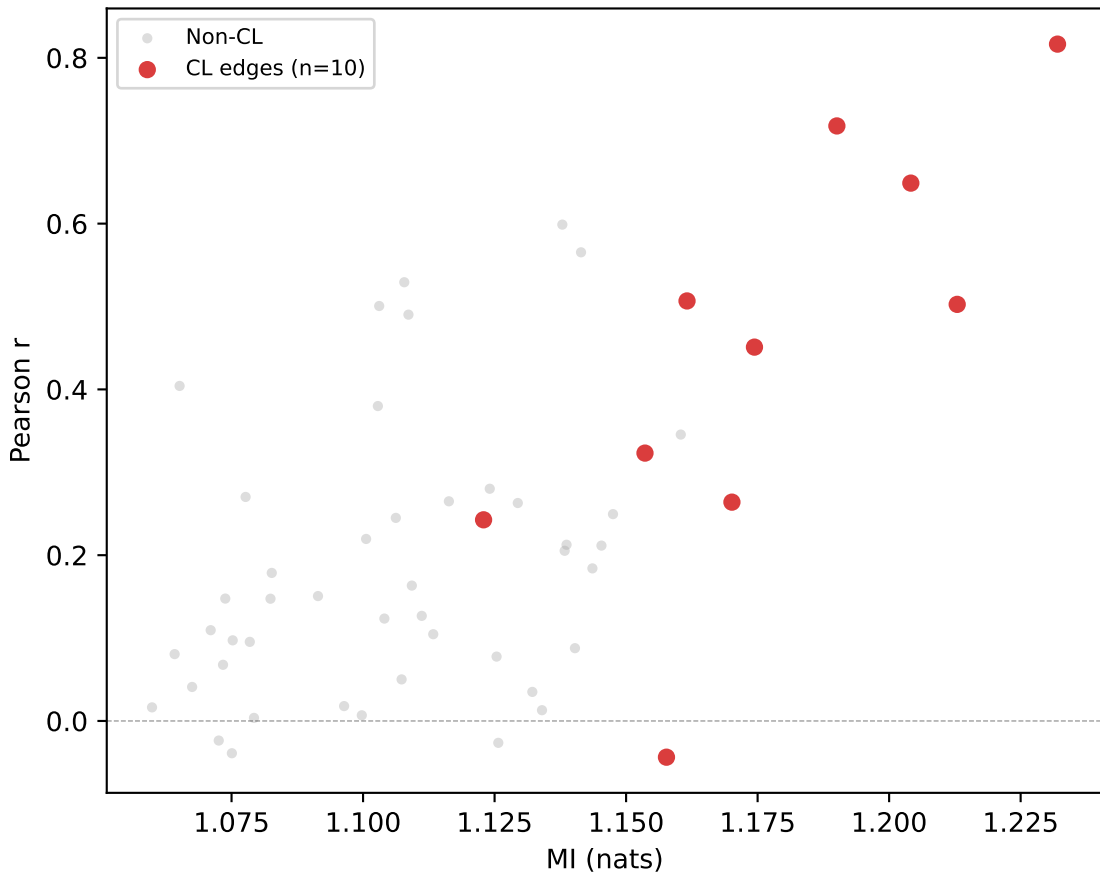
MSC06_func06 — GCSS Motor FC vs MI
