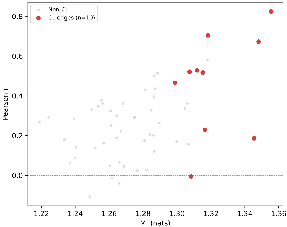
MSC06_func10 — GCSS Motor FC vs MI
