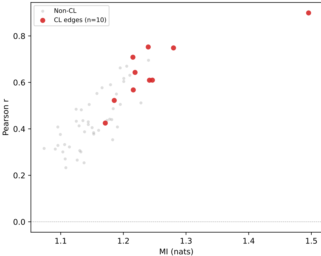
MSC07 func04 — GCSS Motor FC vs MI
