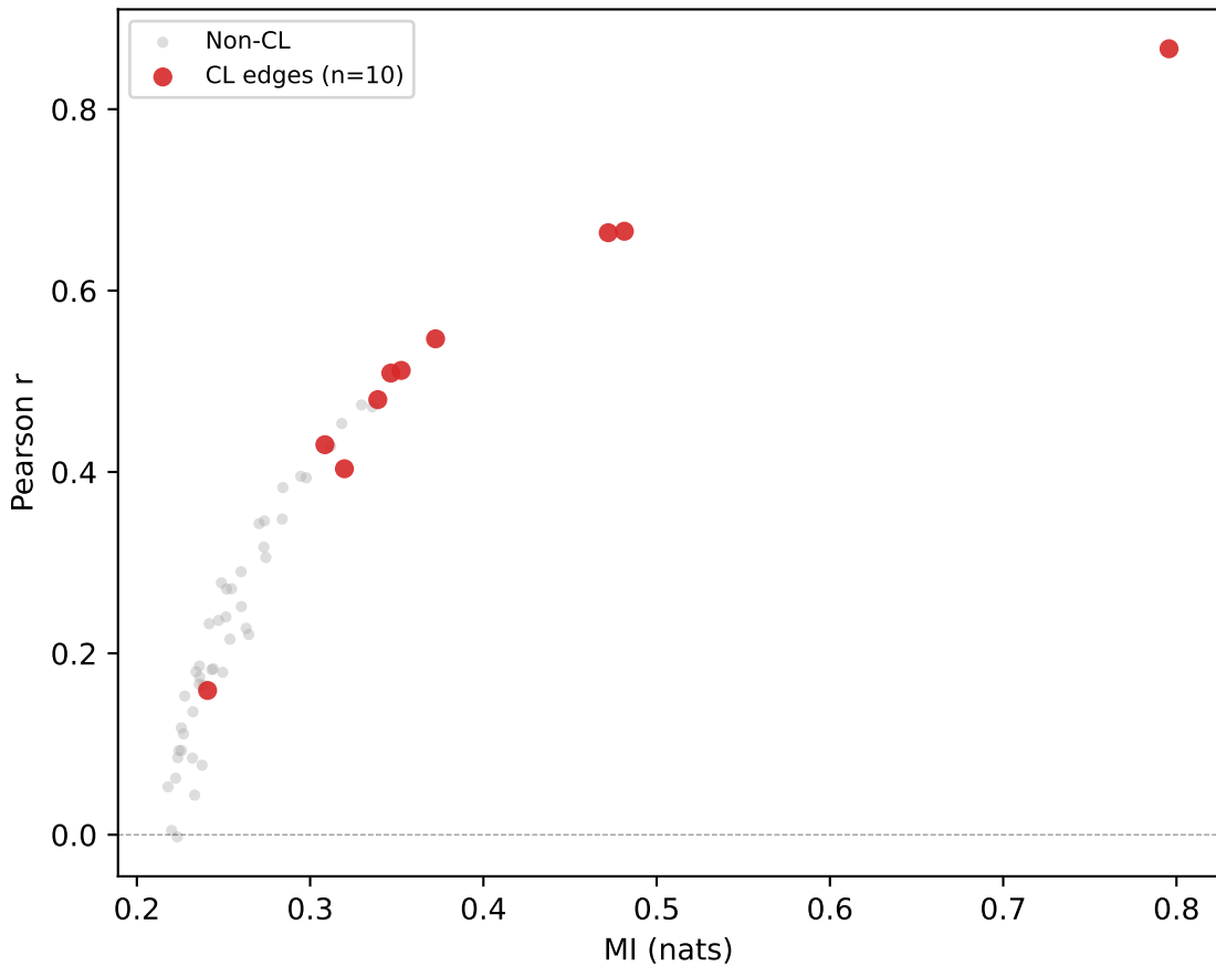
MSC09_all_sessions — GCSS Motor FC vs MI
