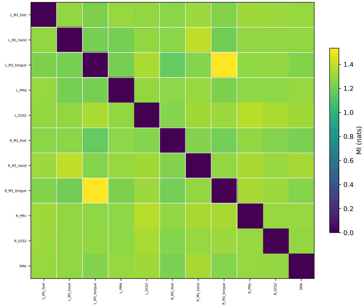
MSC09_func08 — GCSS Motor MI
