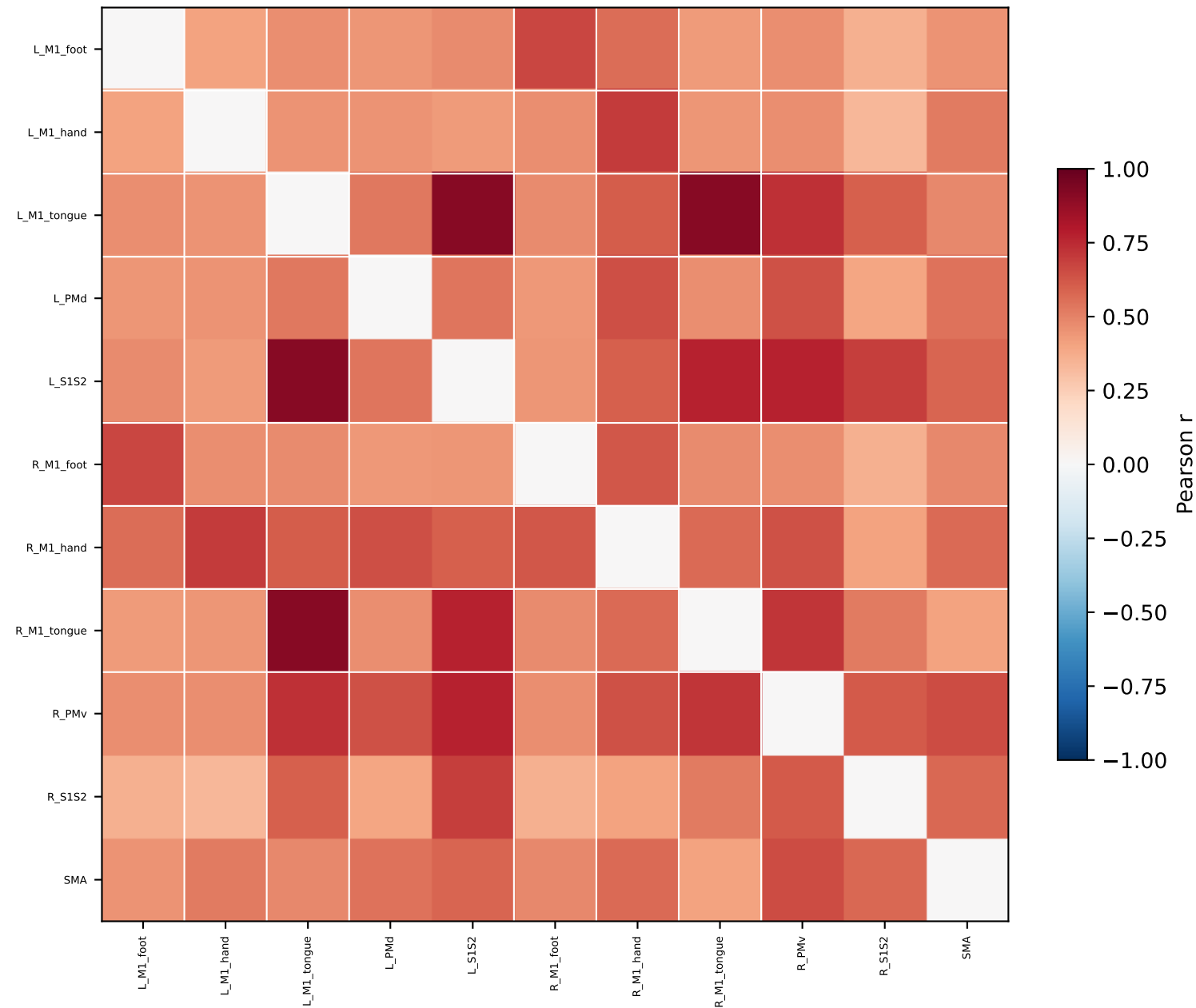
MSC10_func01 — GCSS Motor FC
