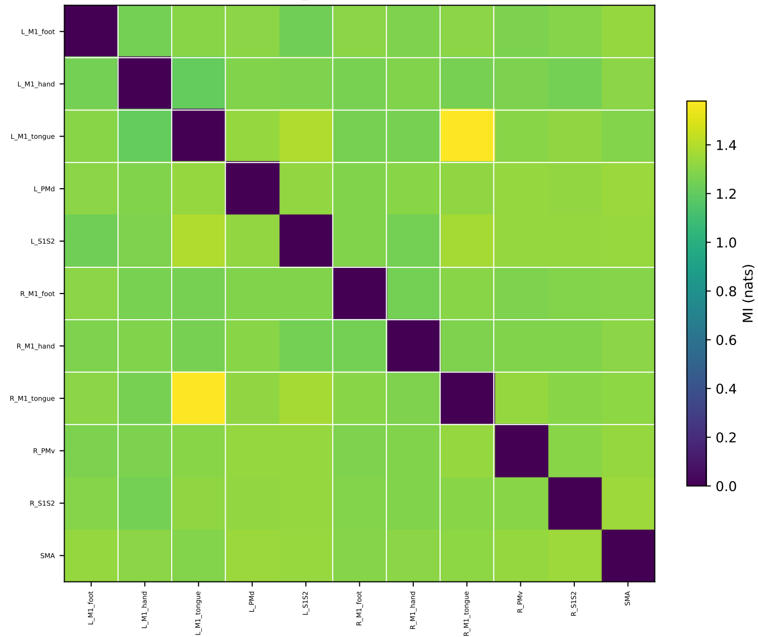
MSC10_func04 — GCSS Motor MI
